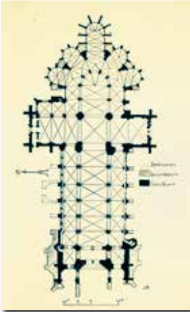
1 PLAN DE LA CATHÉDRALE DE SÉES. En hachuré apparaissent les maçonneries ajoutées à partir du XVI e s. pour renforcer les murs. Les tours de la façade et le mur nord de la nef présentent en effet des défauts de fondations.
